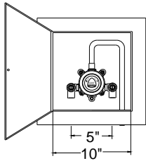
TA-254-LF
