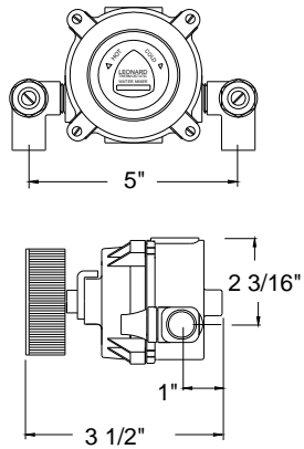
TA-254-LF
